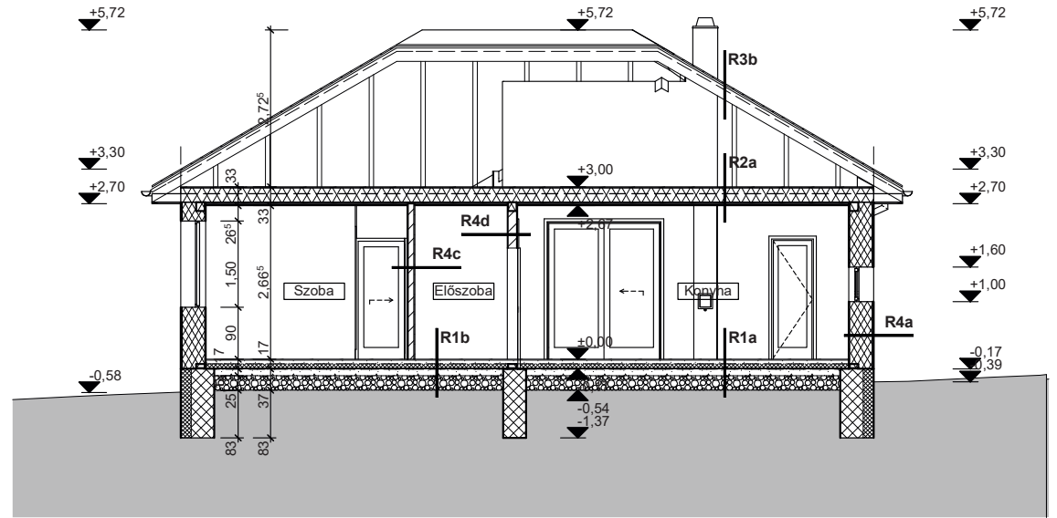
B-B Metszet
