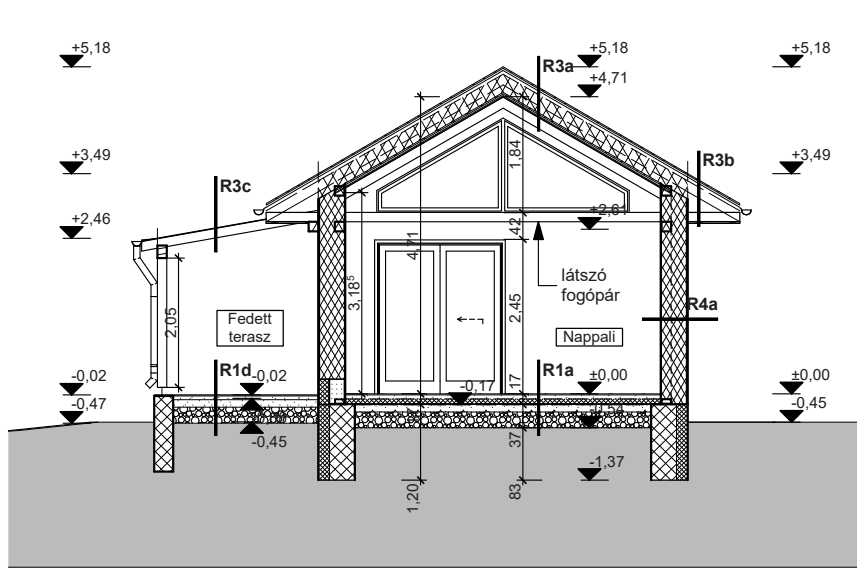
A-A Metszet (1)
